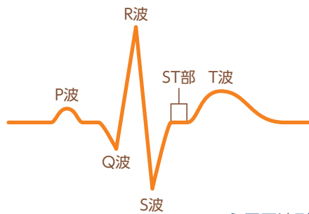
心電図波形
